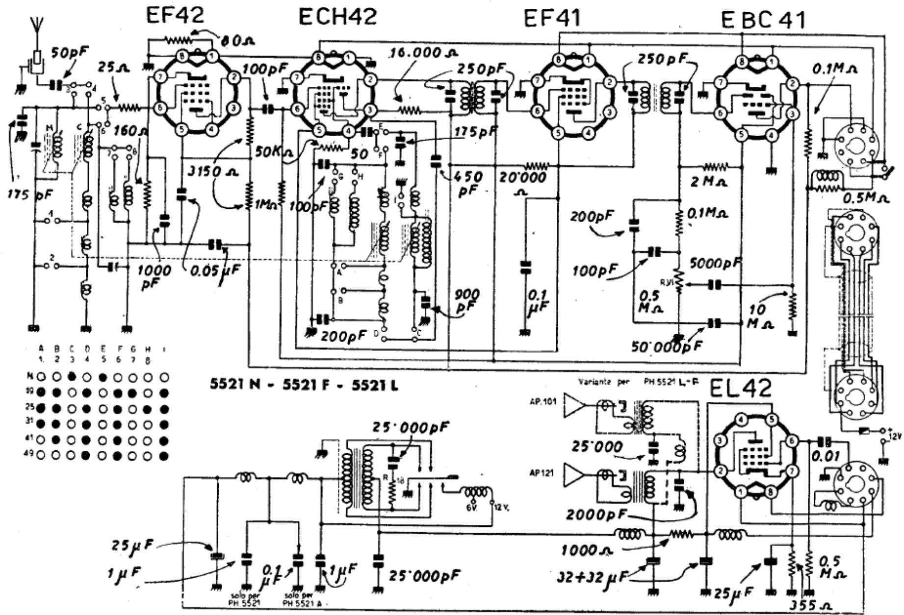
PHONOLA RADIO - AUTORADIO mod. 5521 N-F-L - Sintonia a permeabilità variabile. Gamma OM intera e cinque bande OC espanse a 19, 25, 31, 41 e 49 m. (N = normale, F = Fiat, L = Lancia). MF a 470 kc. Consumo 2,4 A a 12 V cc. Uscita 1,8 W.
